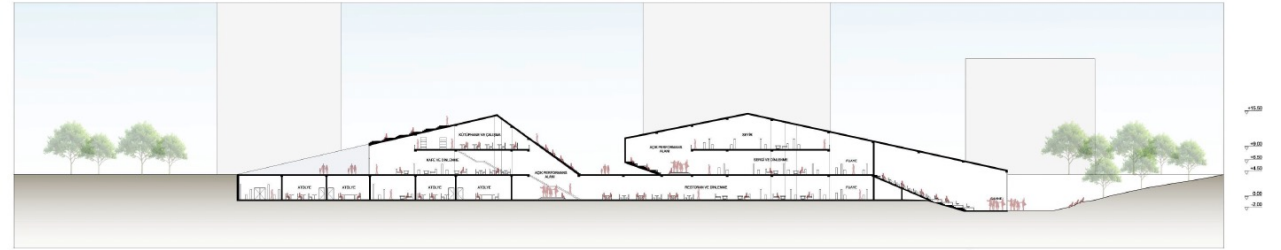
1/200 AA KESİTİ
